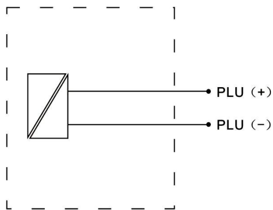
无源型内部示意图
