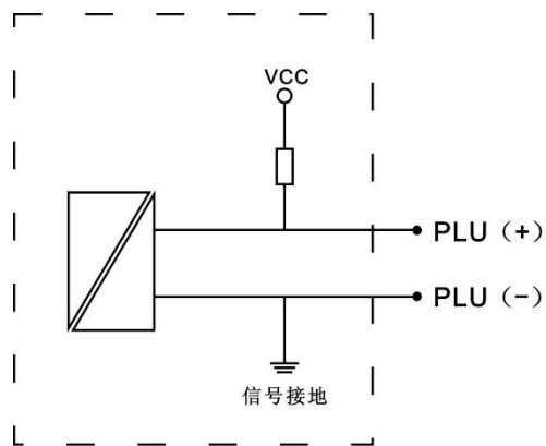
有源型内部示意图
